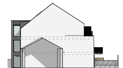
Východní pohled
